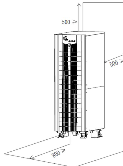
Rys. 3-1. Wymiary zalecanej przestrzeni serwisowej
