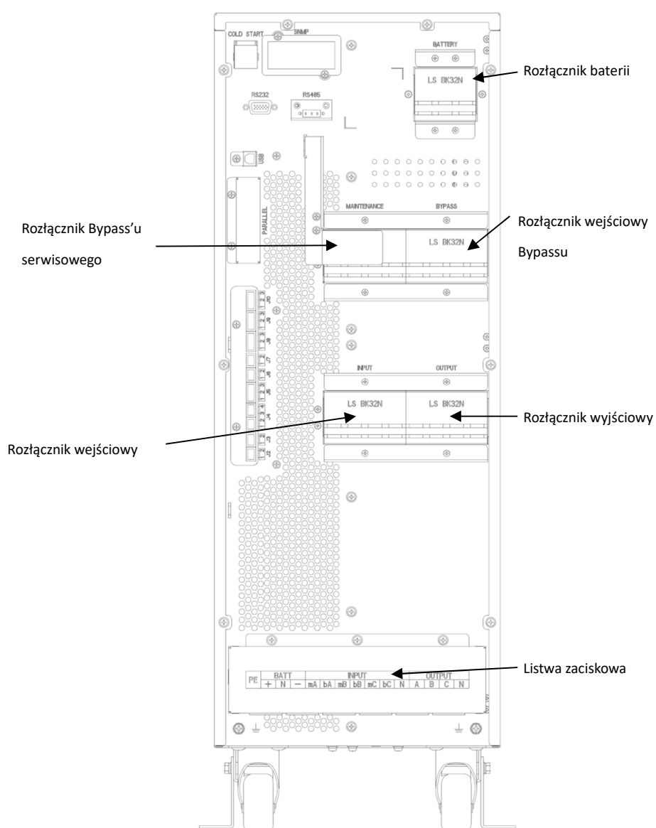
Rysunek 4-1 Rozmieszczenie łączników zasilania w zasilaczu NGS 10-15K
