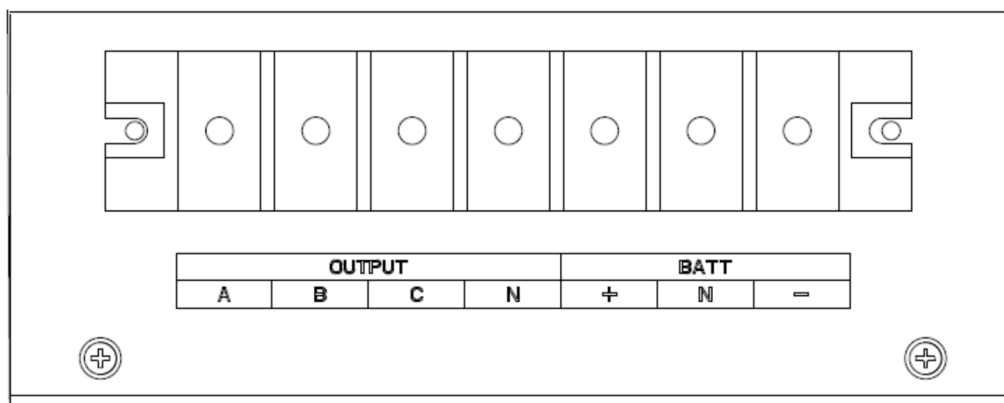
Część lewa listwy zaciskowej
