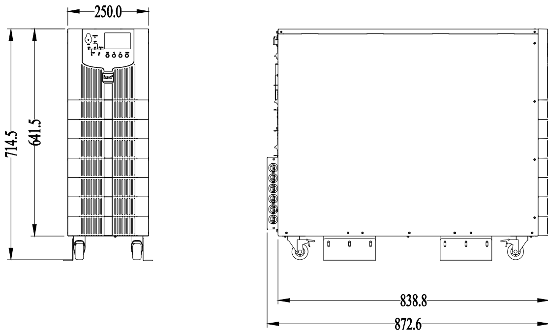
Rysunek 2-2 Widok przód/bok zasilacza UPS NGS 10-15
