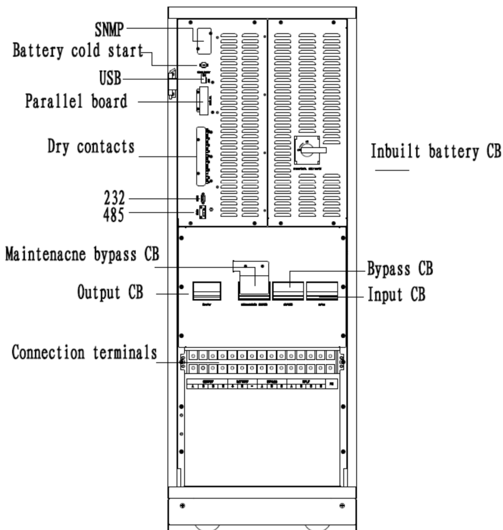
Rysunek 2-8 Widok przedniej ściany zasilacza i podejścia przewodów NGS 40K
