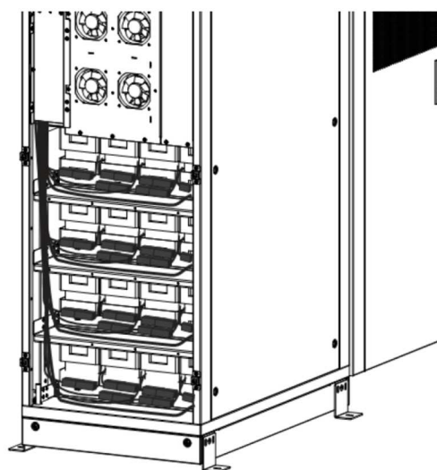
Rysunek 2-12 Widok rozmieszczenia i połączenia baterii zależnie od typu UPS
