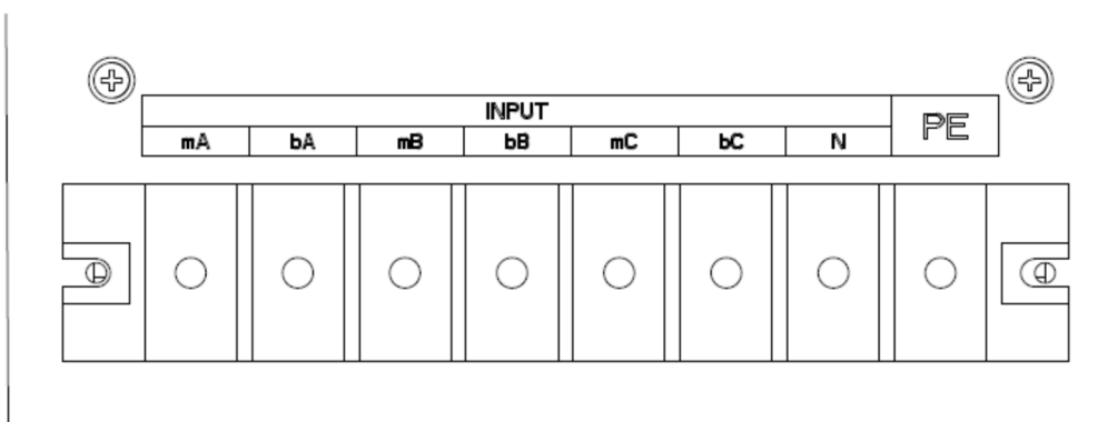
Część prawa listwy zaciskowej
