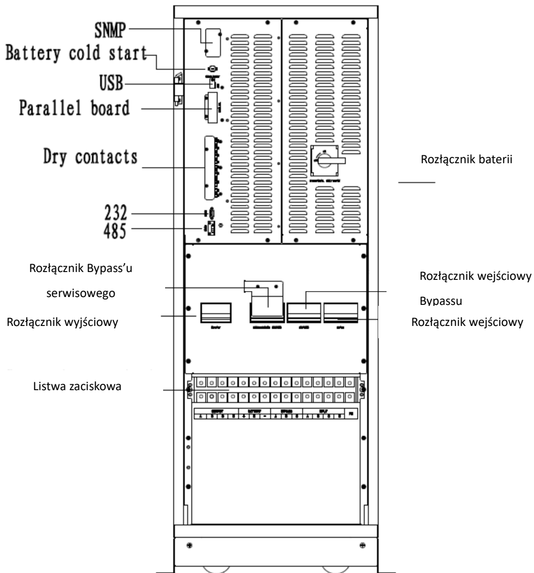
Rysunek 4-3 Rozmieszczenie łączników zasilania w zasilaczu NGS 40K
