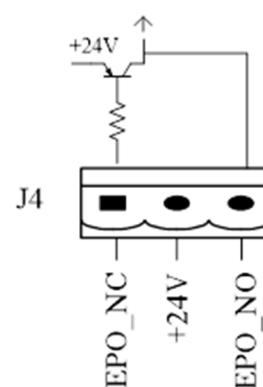
Rysunek 2-16 Interfejs REPO
