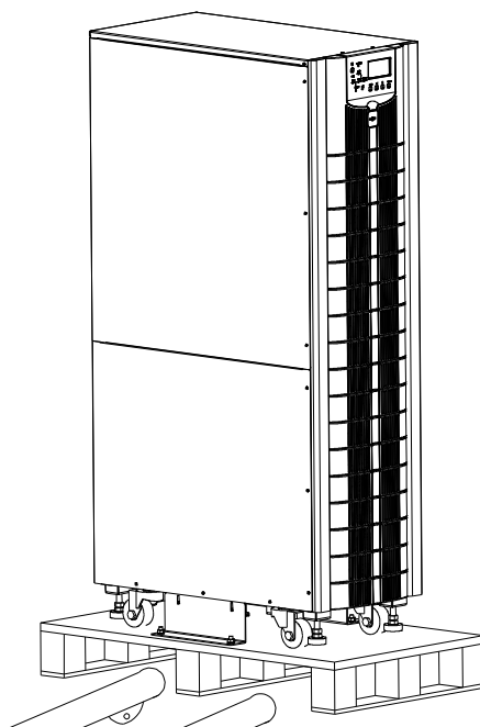
Rysunek 2-1 Widok przykładowego zasilacza po demontażu opakowania
