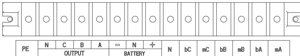
Rysunek 2-10 Widok listwy zaciskowej do podłączenia przewodów NGS 20-30
