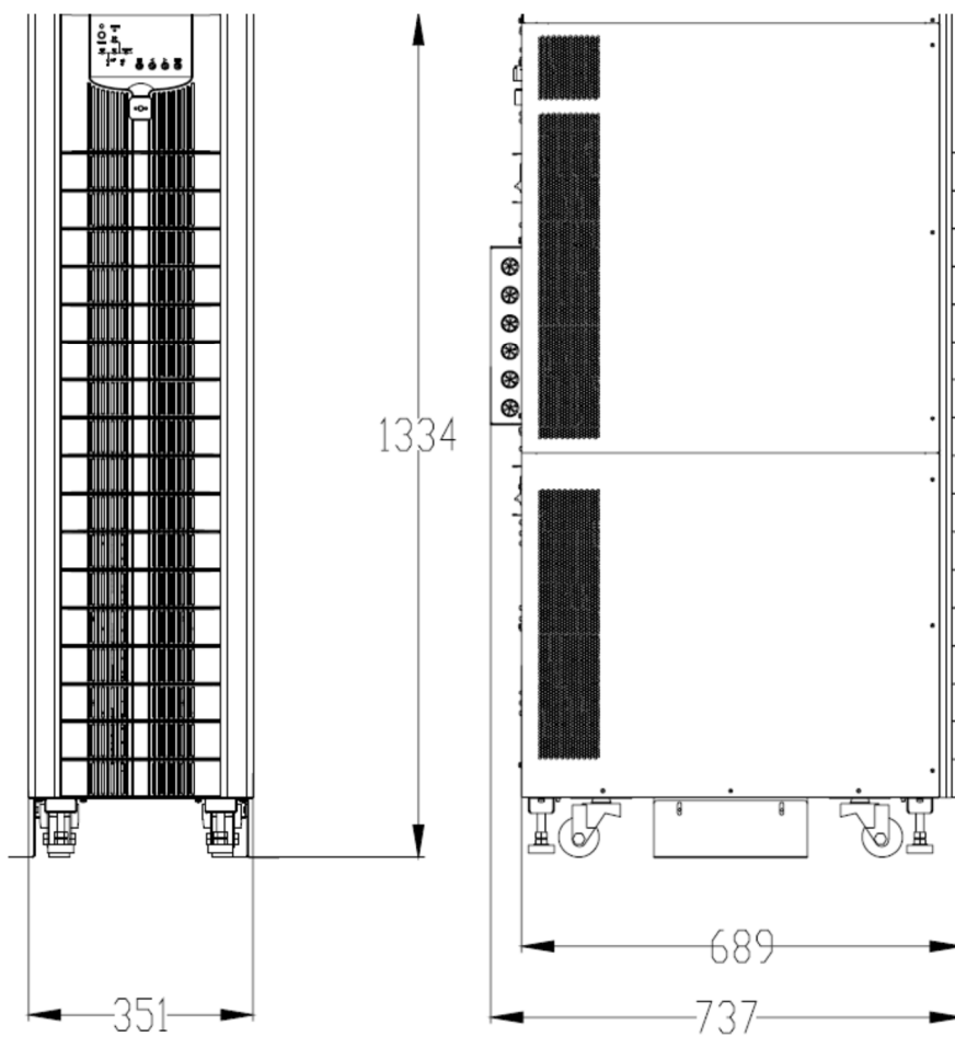
Rysunek 2-2 Widok przód/bok zasilacza UPS NGS 10-15
