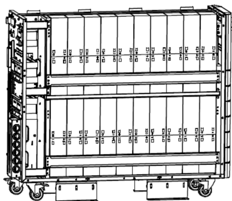
Rysunek 2-12 Widok rozmieszczenia i połączenia baterii zależnie od typu UPS
