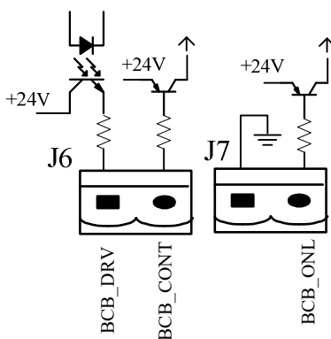
Rysunek 2-17 Interfejs BCB
