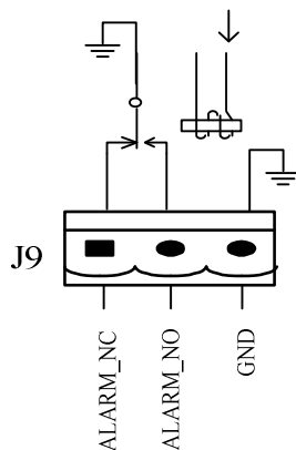
Rysunek 2-19 Interfejs alarmowy
