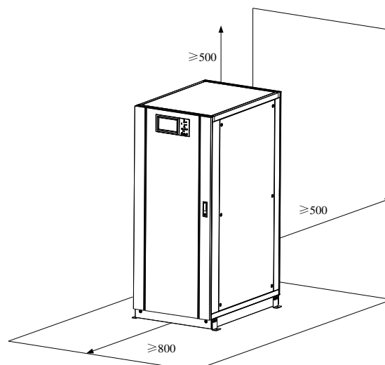
Rys. 3-1. Wymiary zalecanej przestrzeni serwisowej (wymiary w mm)
