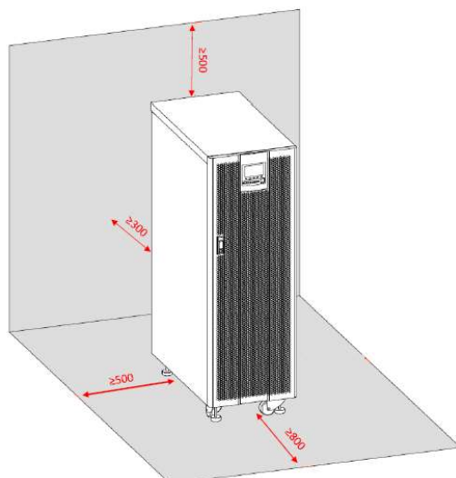
Rys. 3-1. Wymiary zalecanej przestrzeni dla poprawnej wentylacji
